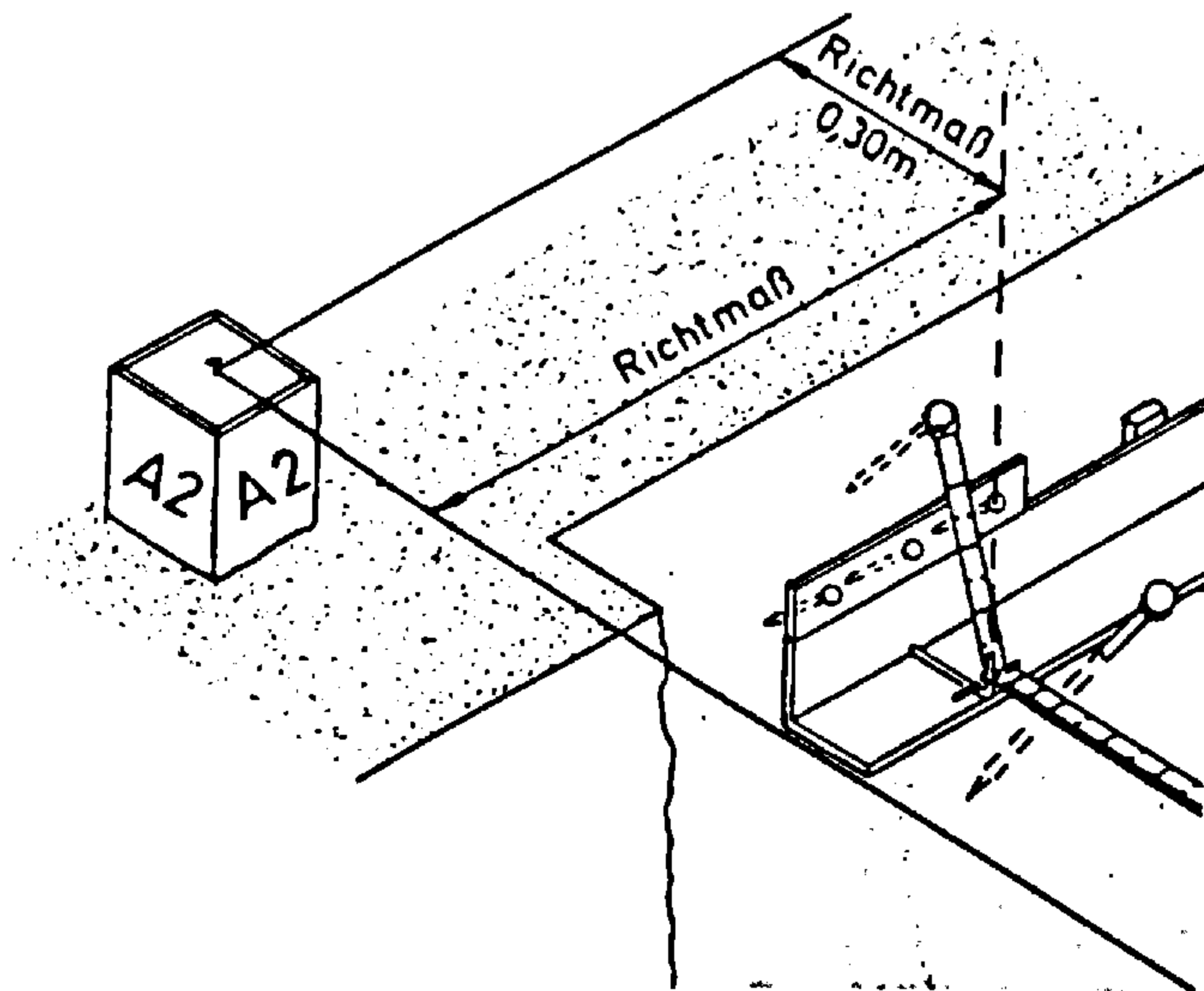
(شكل ١٧) طريقة رفع الموقع
